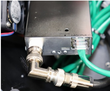
TLC-30PTA-Bに接続/LAN出力からスプリッター-INへ接続
