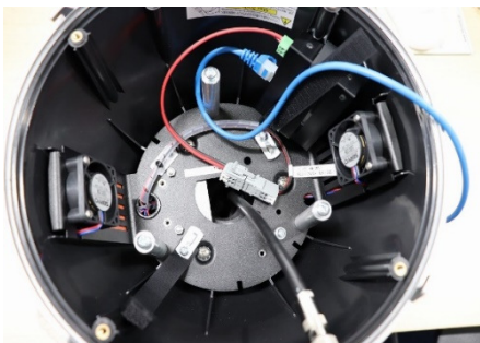
ハウジング内に、同軸1本を配線
